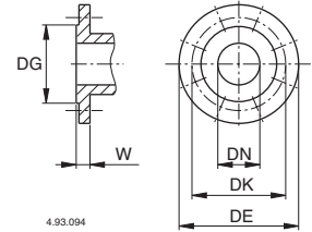
Flanges PN 10, EN 1092-2
